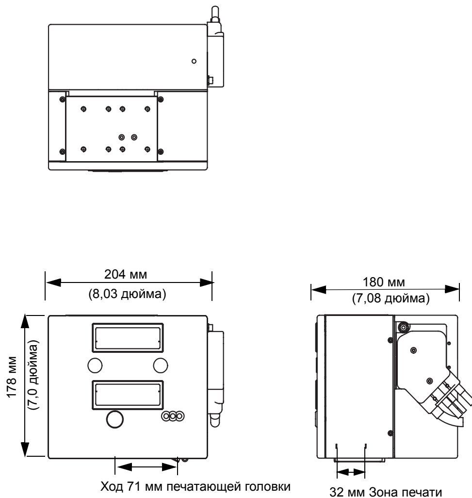
Рис. 7-4: Размеры принтера Videojet DataFlex 6320 32 мм, левостороннего
