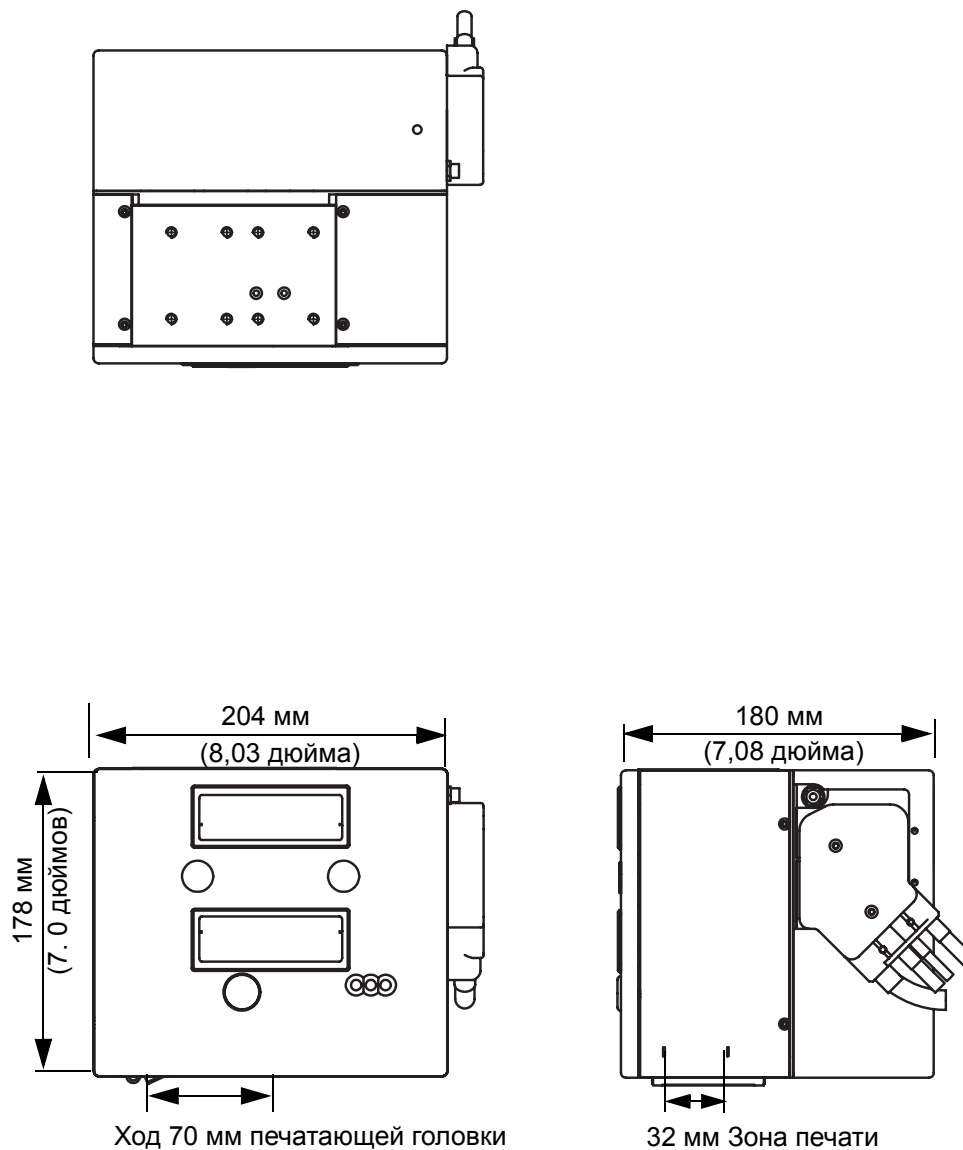
Рис. 7-3: Размеры принтера Videojet DataFlex 6320 32 мм, правостороннего
