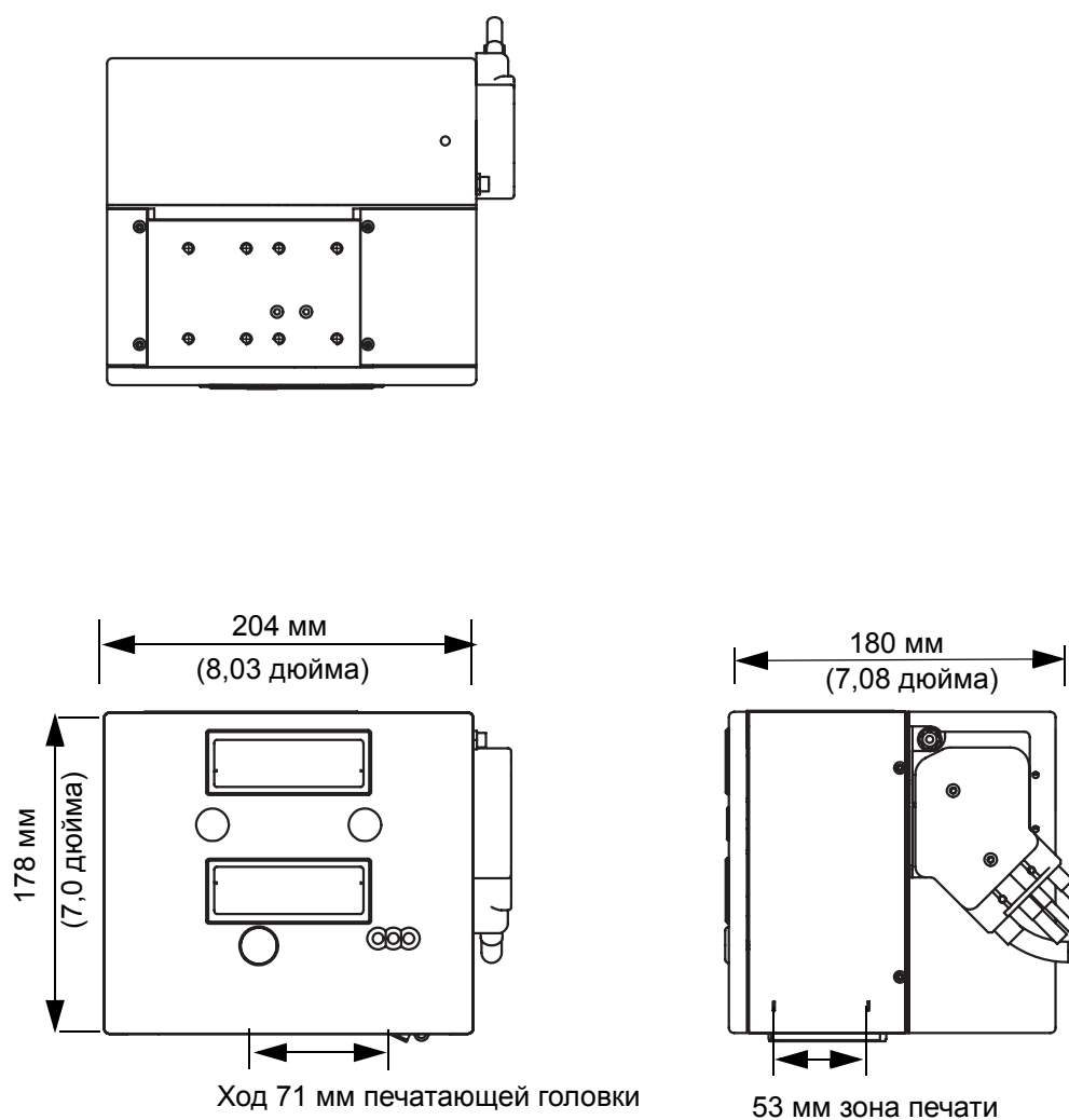
Рис. 7-2: Размеры принтера Videojet DataFlex 6320 53 мм, левостороннего
