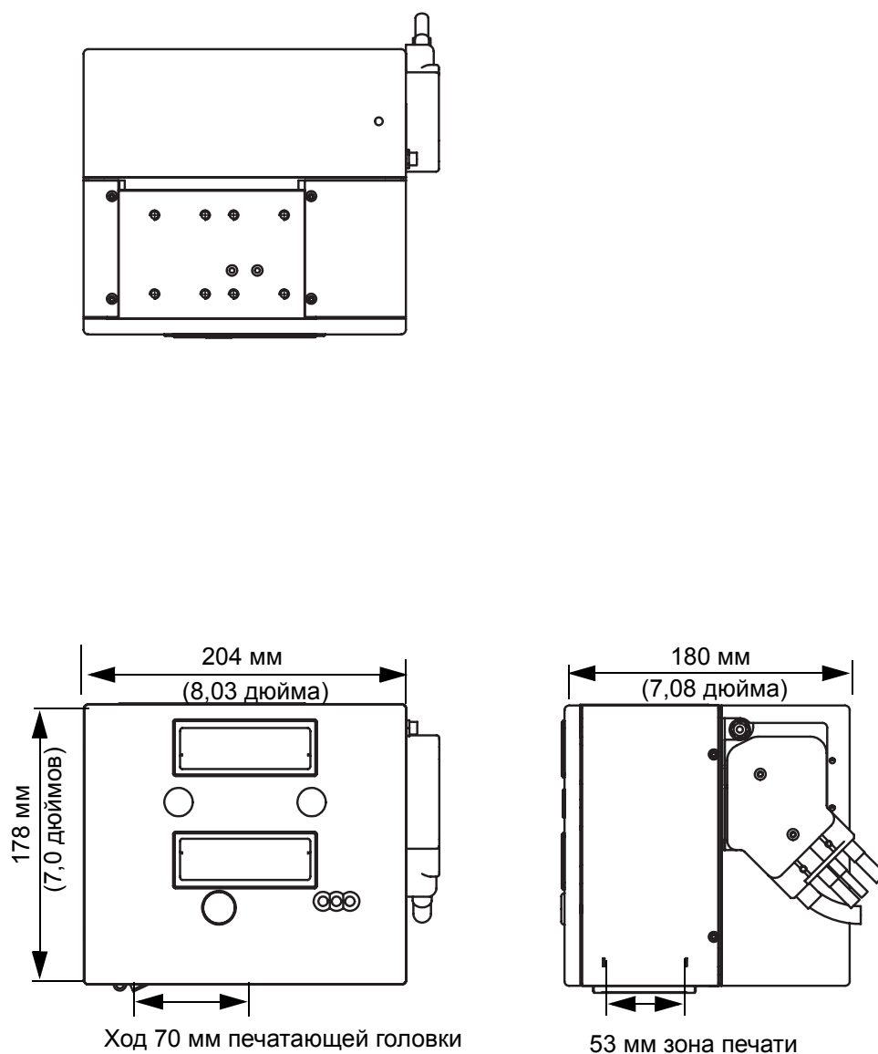
Рис. 7-1: Размеры принтера Videojet DataFlex 6320 53 мм, правостороннего
