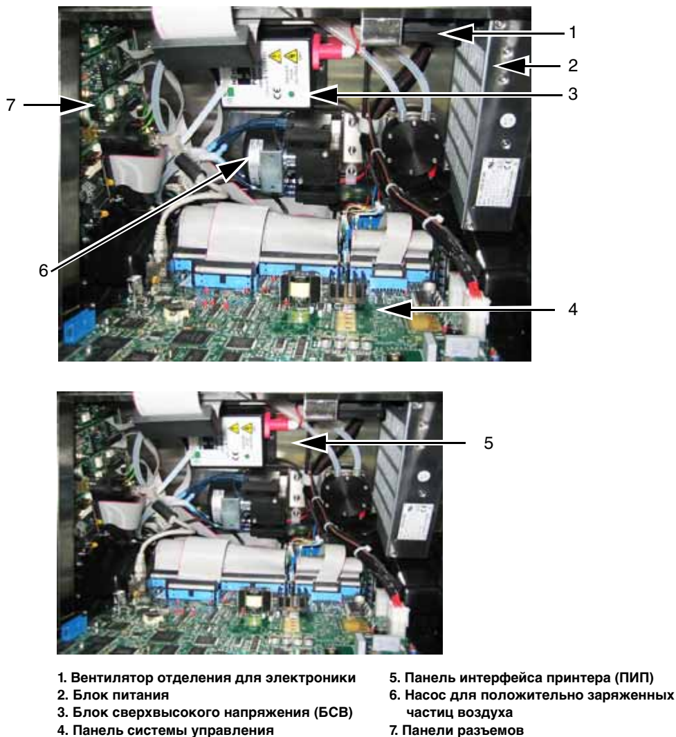
Рисунок 3-4: Отделение для электроники
