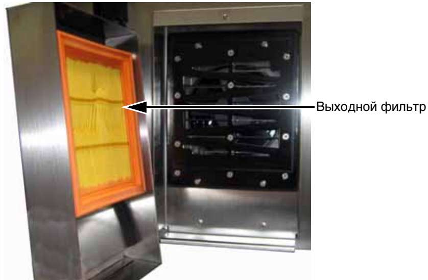
Рисунок 3-10: Выходной фильтр (модель IP65)
